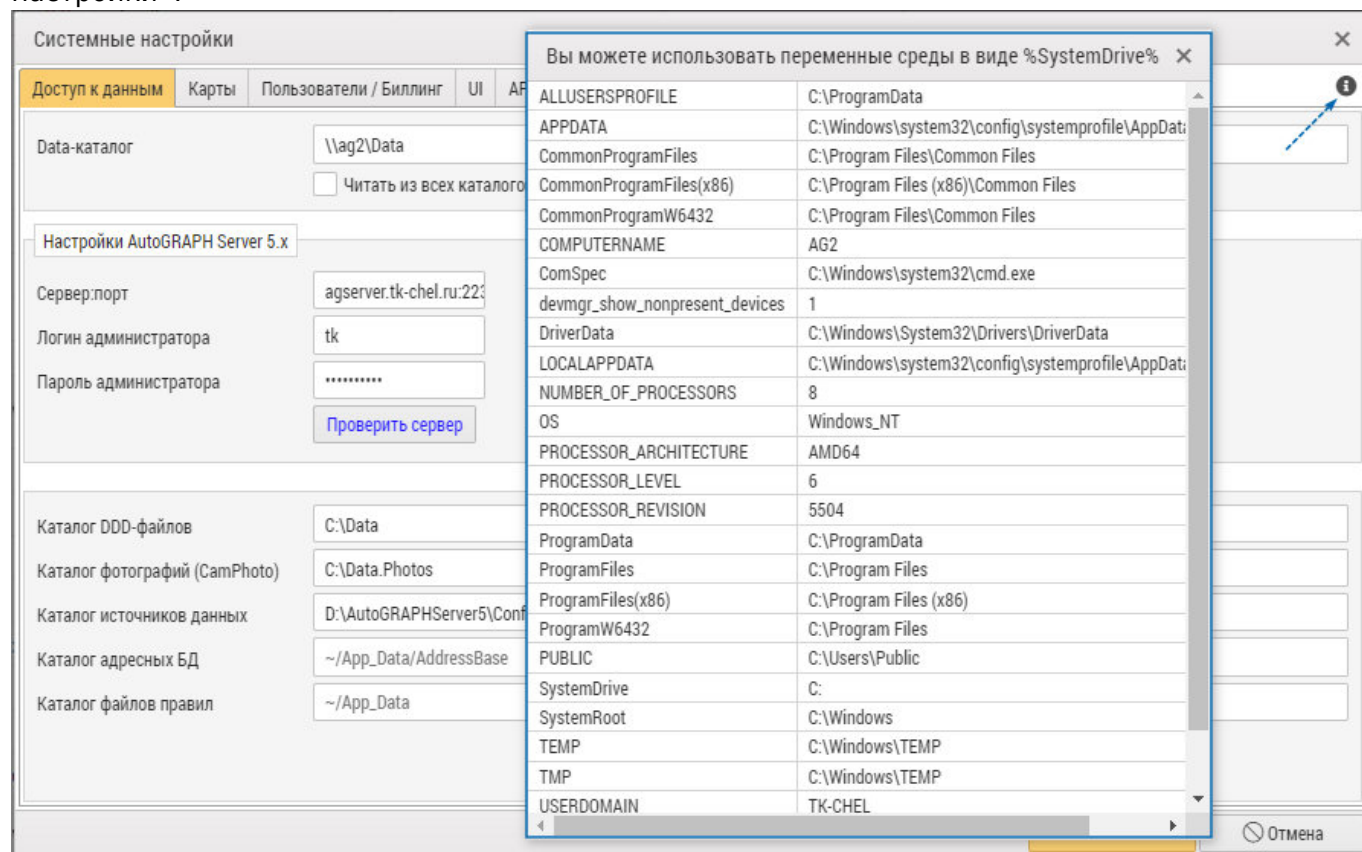
Рис. 3: Переменные среды
