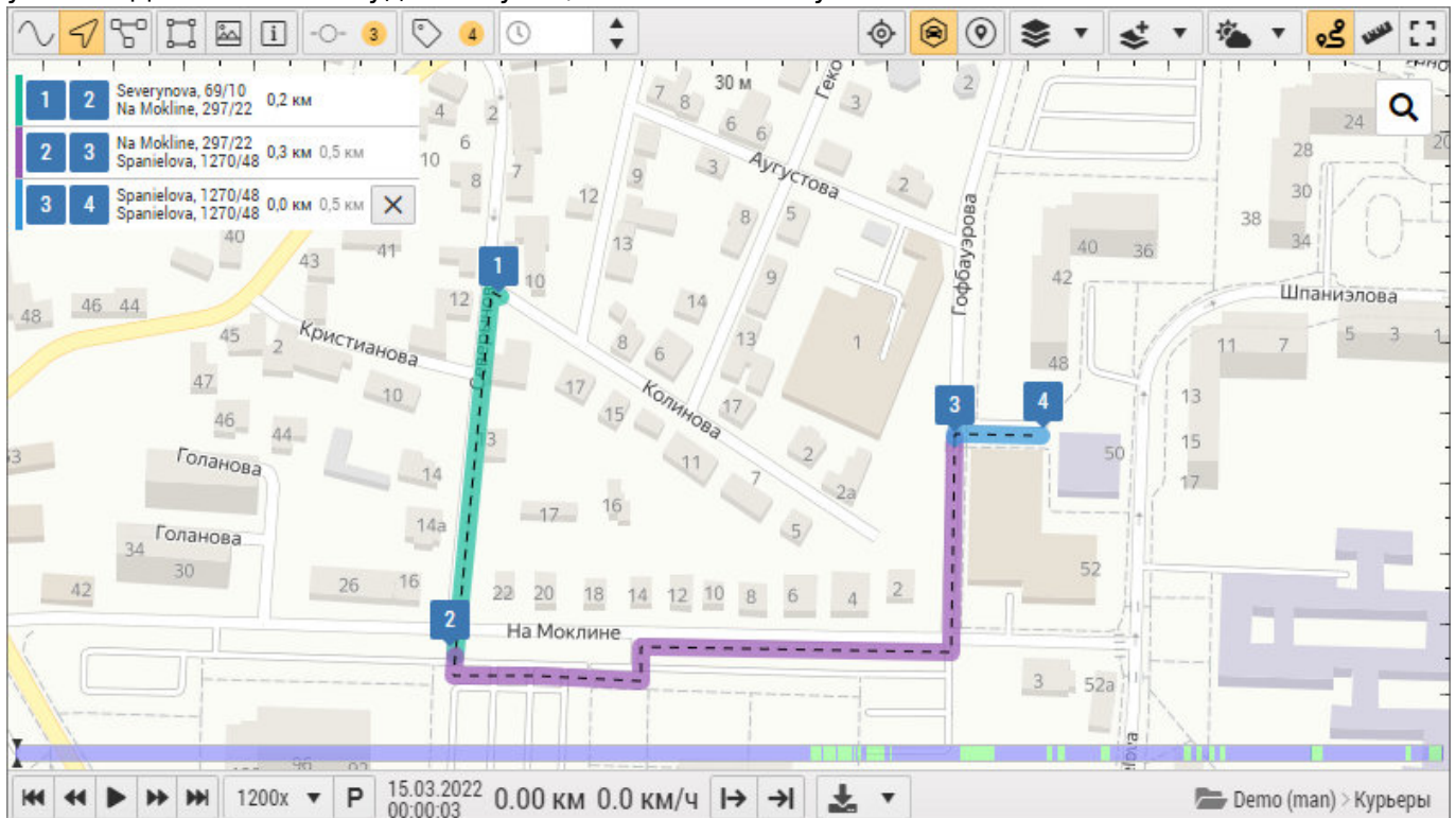
Рис. 6: Построение маршрута
