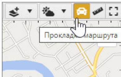
Рис. 5: Построение маршрута
